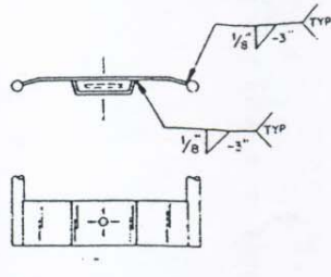
TYP. CABLE BRKT.
